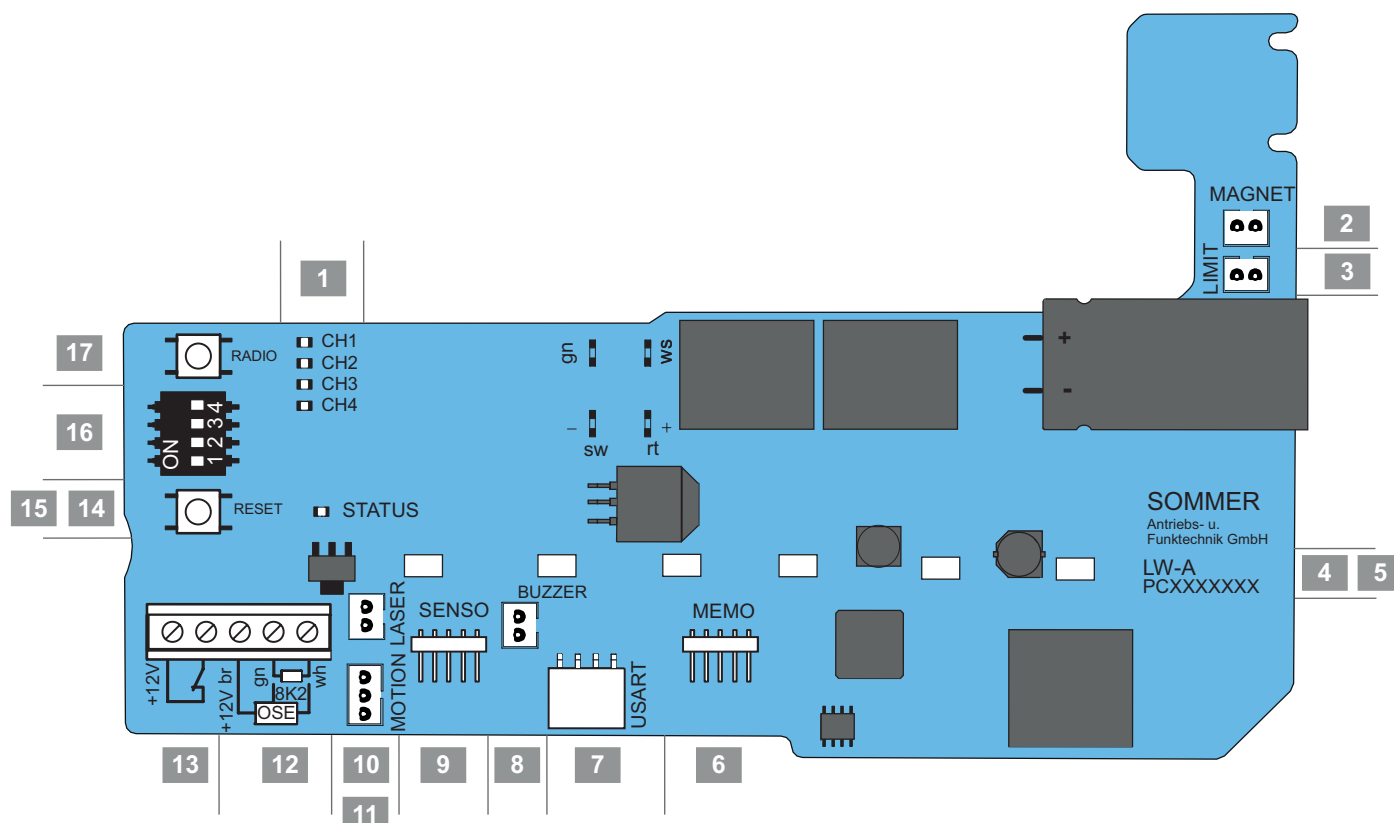
Fig. Løbevognens bundkort, komplet udførelse*
