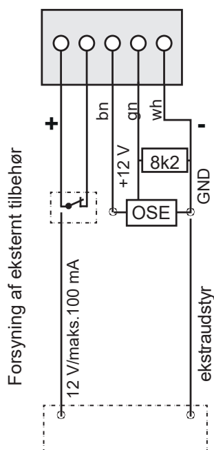
Fig. tilslutningsplan løbevogn
