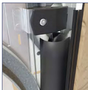
Fjeder inddækninger til RES100EX LODRET
